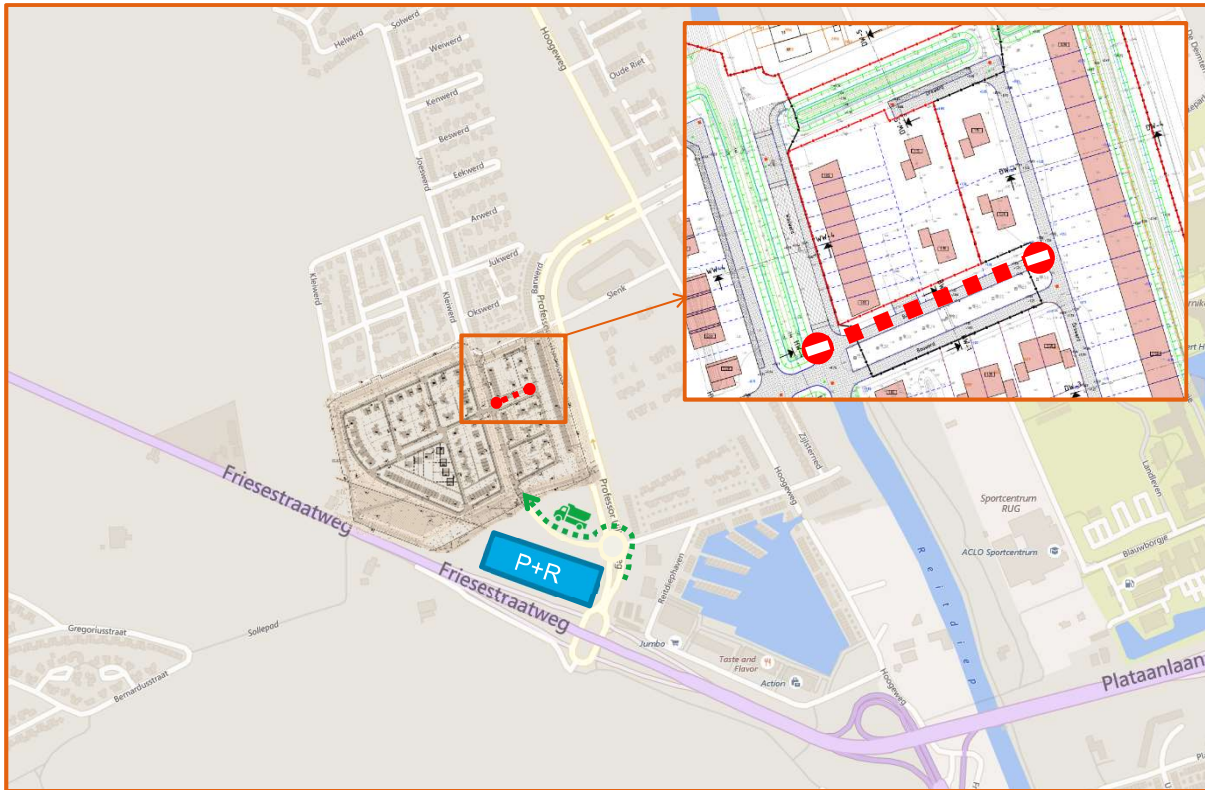
Afbeelding 1 Route bouwverkeer, locatie P+R en scheiding bouwverkeer/schoolverkeer
